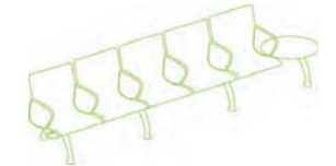
S5G11 5 seater + 1 table OH 800 OW 3210 OD 620 SH 415
