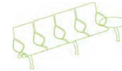
S4G11 4 seater + 1 table OH 800 OW 2665 OD 620 SH 415
